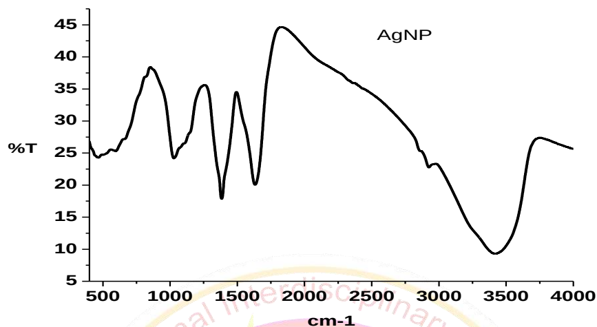
Fig. 4 :FT-IR spectra of AgNP
